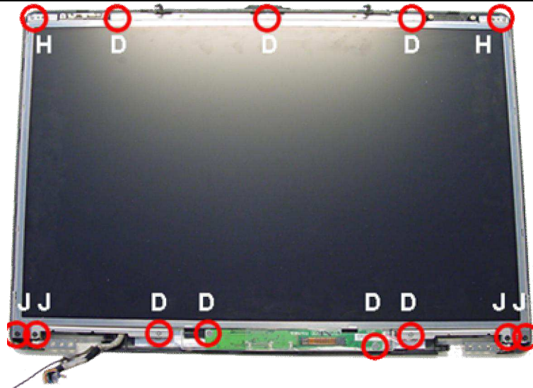
Fig. 15 LCD display panel.
