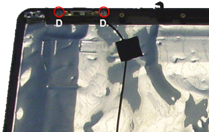
Fig. 19 Wireless antenna.
