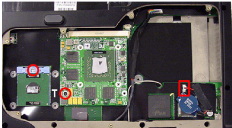
Fig. 7 Remove VGA module and CPU.
